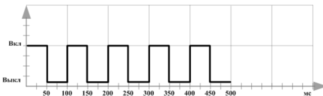
Рис. 10.3. Индикация считывания ключа
