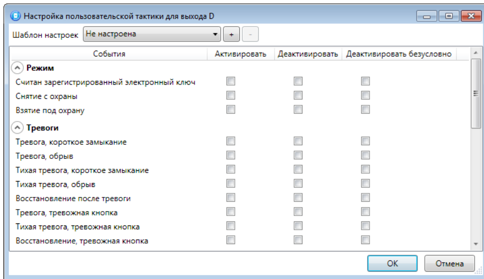
Рис. 5.27. Настройка пользовательской тактики для выхода
