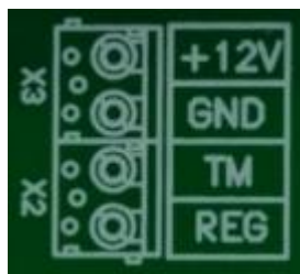
Рис. 7.3. Маркировка выходов и схема подключения считывателя STEMAX RFID
