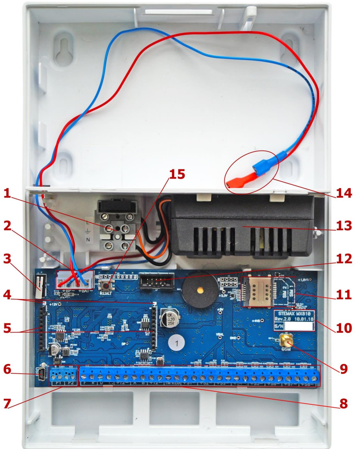
Вид контроллера со снятой крышкой
