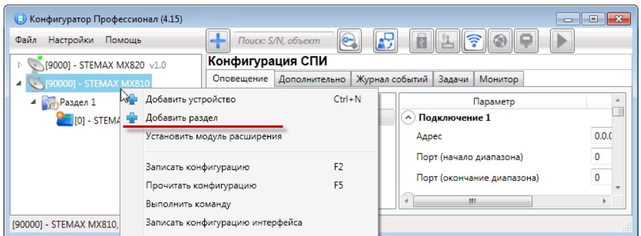
Рис. 5.16. Добавление к контроллеру СКП в качестве раздела
