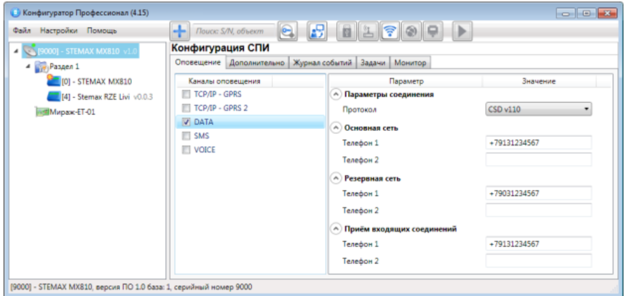
Рис. 5.8. Параметры канала DATA
