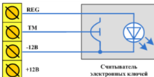
Рис. 7.1. Схема подключения считывателя Touch Memory
