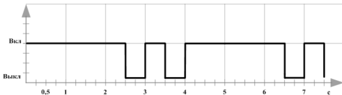
Рис. 10.5. Индикация режима На охране со шлейфом в состоянии Тревога и режима На охране с аварией
