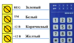
Рис. 10.4. Схема подключения кодовой панели Мираж-КД и пульта управления ПУ-ТМ ВОРС Стрелец
