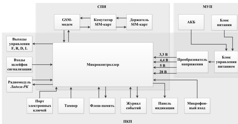
Рис. 3.1. Функциональная схема контроллера Мираж-GSM-A4-02
