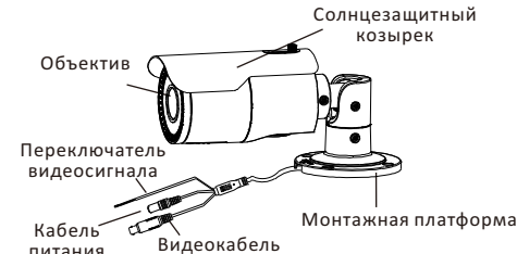
Рисунок 1-2 Внешний вид камеры II типа
